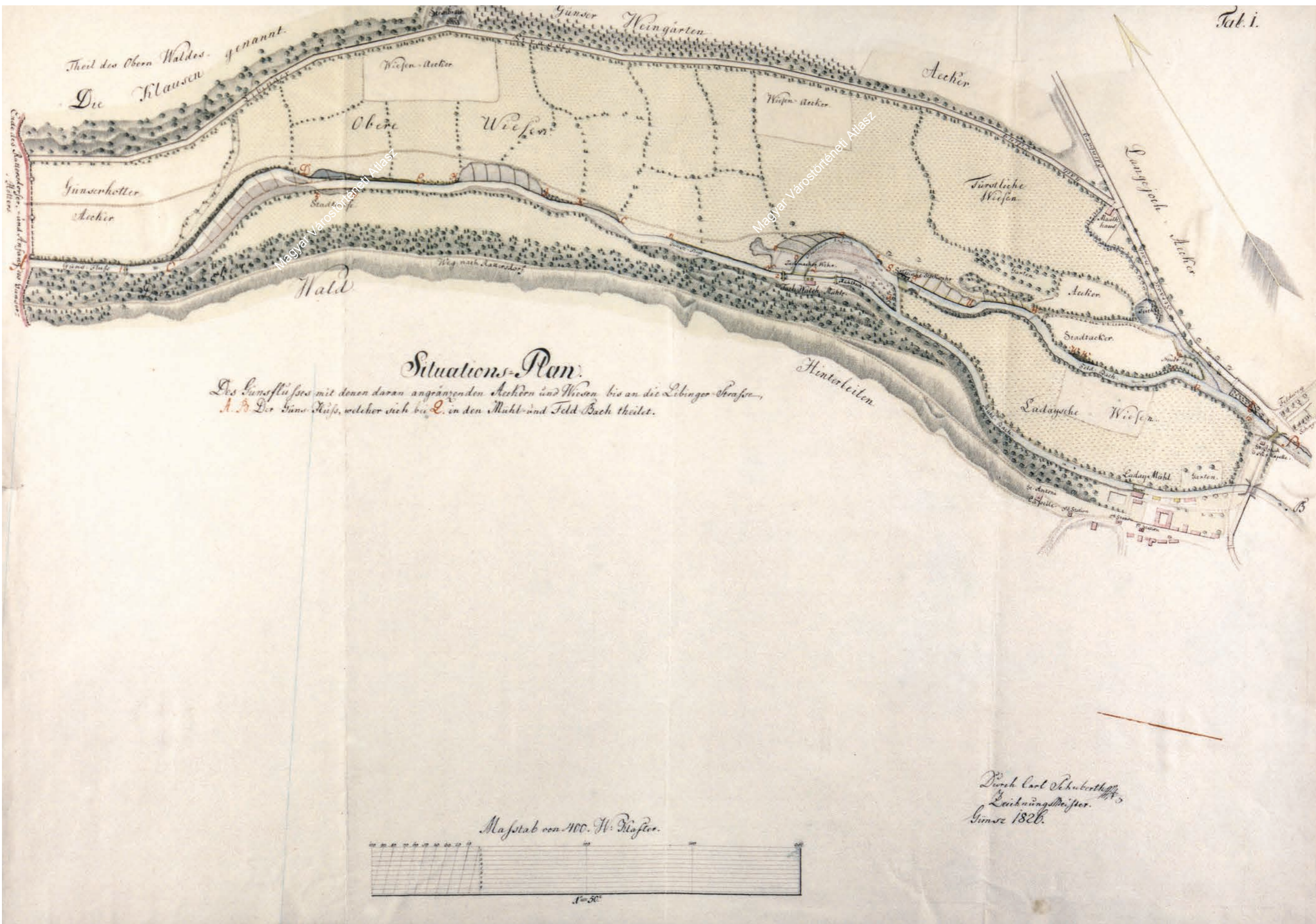
C.1.3.1 A Gyöngyös-patak helyszínrajza. I. Tab., Karl Schubert, 1826 C.1.3.1 Site plan of the Gyöngyös Stream Tab. I, Karl Schubert, 1826
